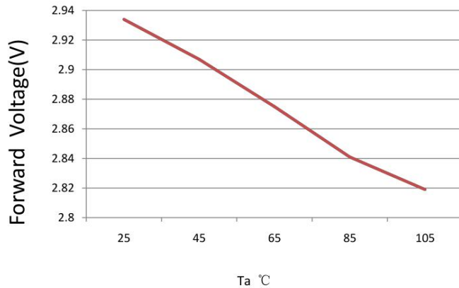
电压与温度曲线:
